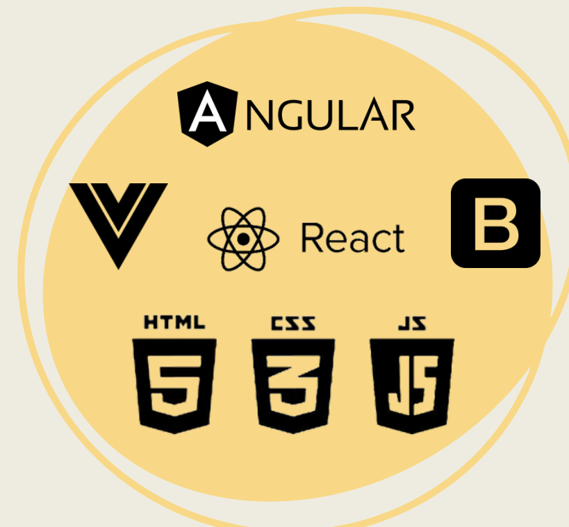
Web Frontend
